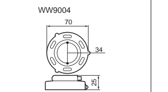
WW9004 標準価格 135円 税別 セードホルダ
